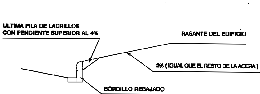
SECCION A-A
